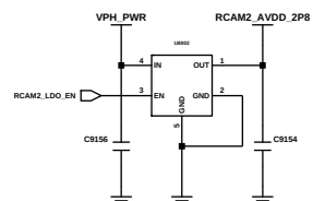
RCAM2_AVDD
